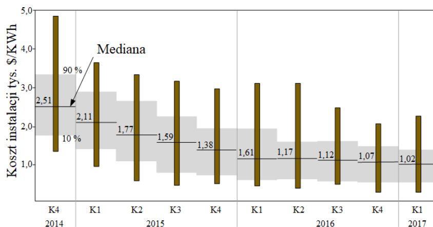
Rys. 7. Koszt instalacji akumulatorów Li-ion (w zrealizowanych projektach) z zaznaczeniem mediany [18]
