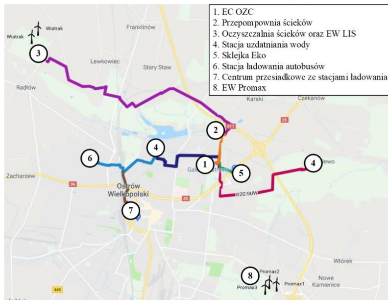
Rys. 10. Własna sieć SN klastra ORE
