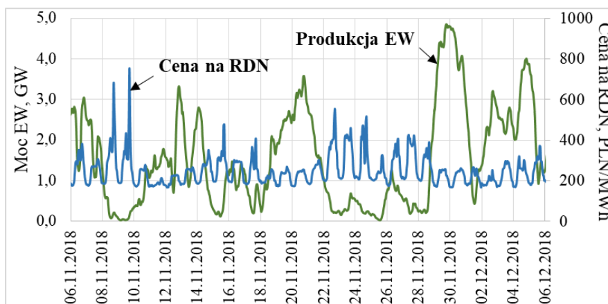
Rys. 6. Porównanie produkcji polskich elektrowni wiatrowych z ceną RDN (06.11.2018 – 06.12.2018) [15]
