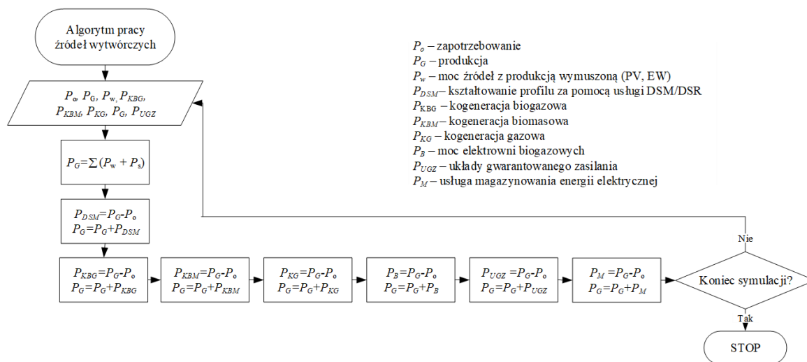
Rys. 11. Kaskadowy algorytm bilansowania klastra ORE
