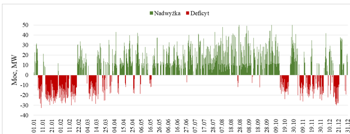
Rys. 12. Profil niezbilansowania klastra ORE
