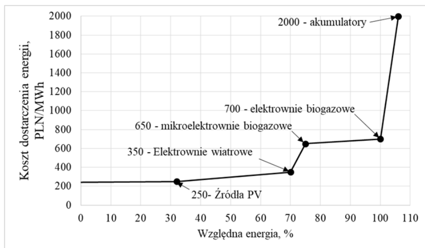
Rys. 6. Koszty krańcowe dostarczania energii w elektroprosumeryzmie dla modelu 3; średnioroczny koszt: 421 PLN/MWh
