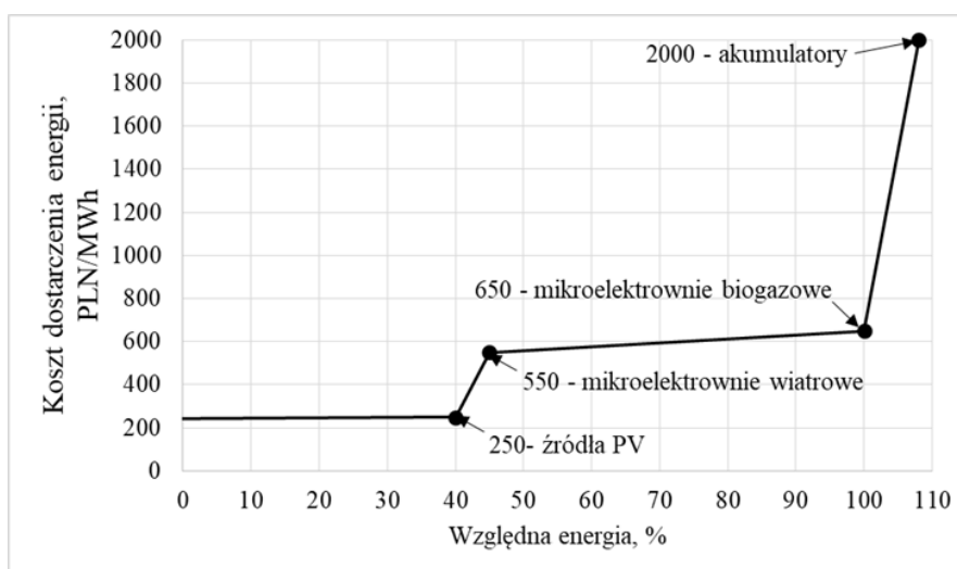
Rys. 4. Koszty krańcowe dostarczenia energii w elektroprosumeryzmie dla modelu 1; średnioroczny koszt: 485 PLN/MWh
