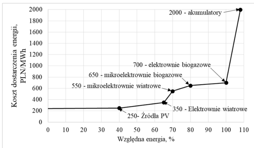
Rys. 5. Koszty krańcowe dostarczania energii w elektroprosumeryzmie dla modelu 2; średnioroczny koszt: 420 PLN/MWh
