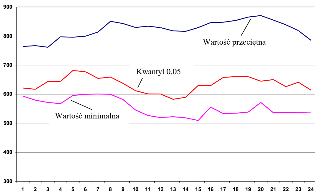
Rys. 3.11. Dynamiczna obciążalność linii z przewodami AFL-240 mm 2 w poszczególnych godzinach doby w okresie zimowym
