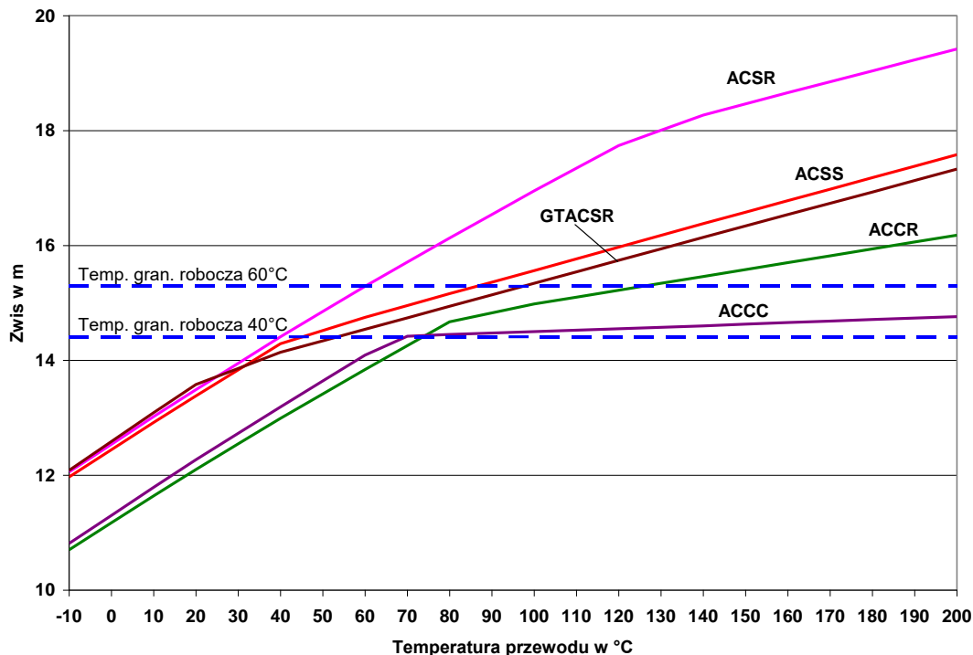
Rys. 3.20. Porównanie zwisów przewodu AFL-8 402/454 mm 2 ze zwisami równoważnych przewodów wysokotemperaturowych w przęśle 450 m z naciągiem podstawowym 46750 N
