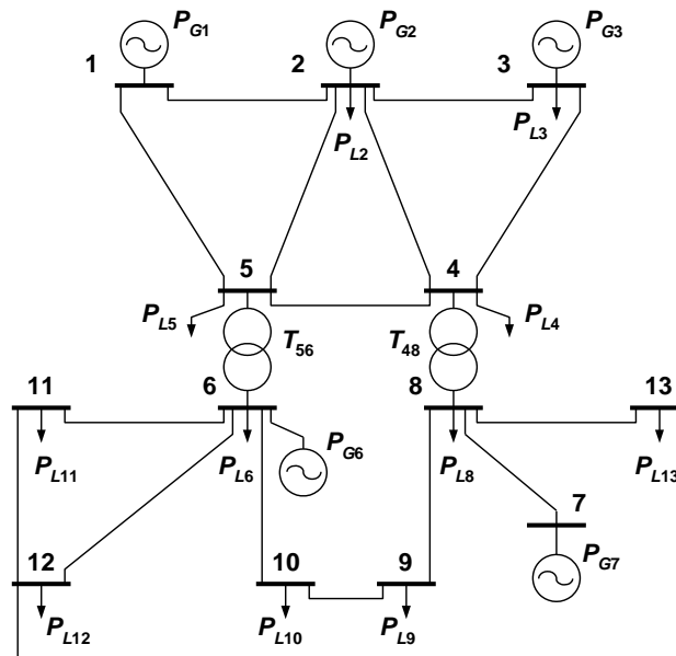
Rys. Z.4.1. Schemat systemu testowego
