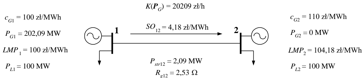
Rys. Z. 5. Wpływ strat mocy czynnej na krótkookresowe ceny węzłowe LMP i stawkę punkt-punkt opłaty rynkowej
