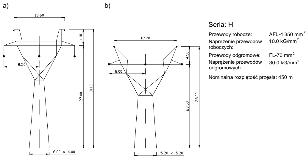
Rys. 3.19. Sylwetki słupów kratowych dwóch starych polskich linii 220 kV z przewodami roboczymi AFL-8 402/454 mm 2 i AFL-4 350 mm 2 : a) przelotowy; b) odporowo-narożny ONII
