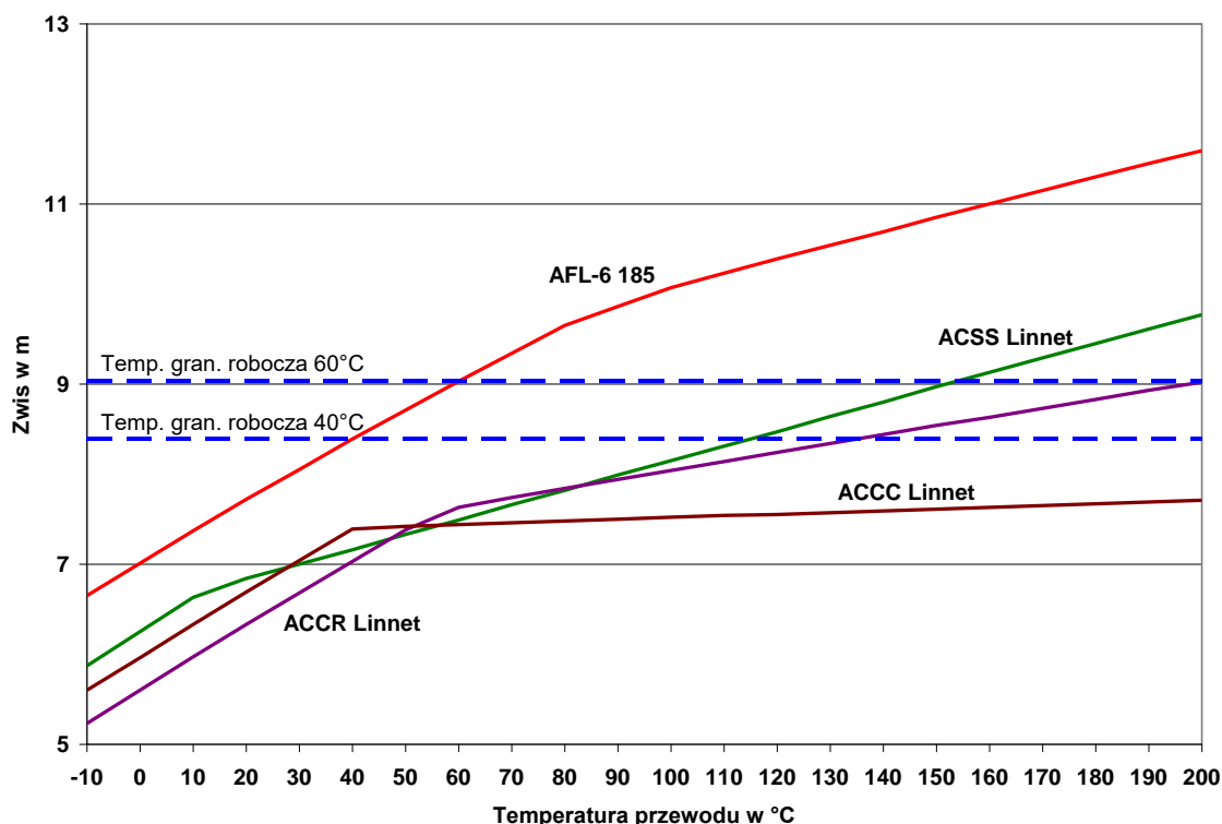
Rys. 3.18. Porównanie zwisów przewodu AFL-6 185 mm 2 ze zwisami równoważnych przewodów wysokotemperaturowych w prześle 300 m z naciągami podstawowymi 21550 N
