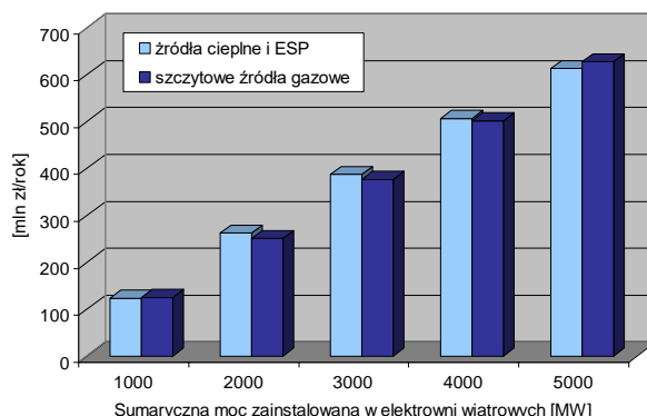
Rys. 4. Roczne koszty zakupu rezerwy godzinowej w elektrowniach ciepłych i szczytowo-pompowych oraz w źródłach szczytowych z turbinami gazowymi
