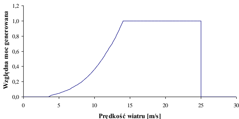
Rys. 3.13. Charakterystyka mocy generowanej przez elektrownię wiatrową.
