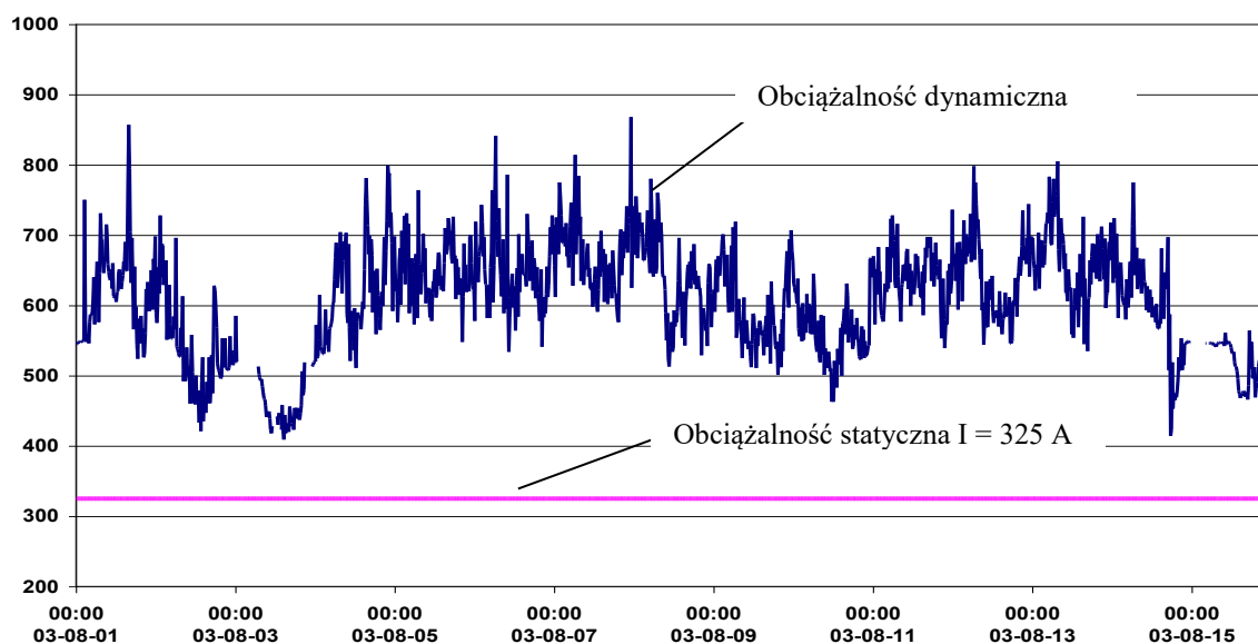
Rys. 3.1. Obciążalność wybranej linii 110 kV z przewodami AFL-6 240 mm 2 w zmiennych warunkach atmosferycznych
