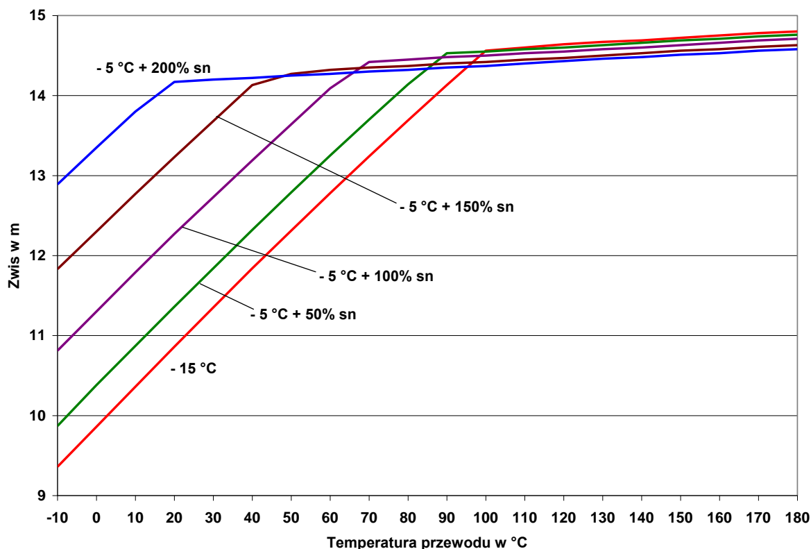
Rys. 3.21. Niestabilność zwisu przewodu ACCC/TW Stockholm w przejście o rozpiętości 450 m po przejściu zimą przez różne obciążenia maksymalne
