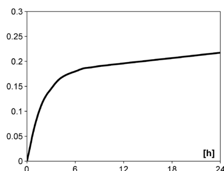
Rys. 4. Odchylenie standardowe błędu prognozy generacji pojedynczej farmy wiatrowej (odniesione do 1 MW mocy zainstalowanej) w zależności od długości horyzontu prognozy [0]
