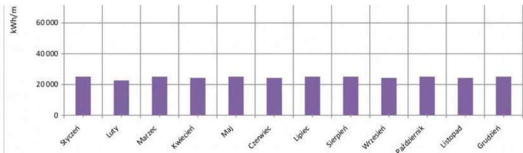
Rys. 11. Przykładowy profil zapotrzebowania na energię do podgrzewu wody basenu całorocznego.
