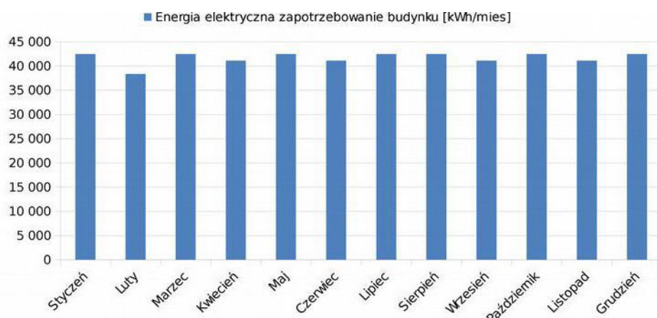
Rys. 15. Przykładowy rozkład zapotrzebowania na energię elektryczną w obiekcie w skali roku.
