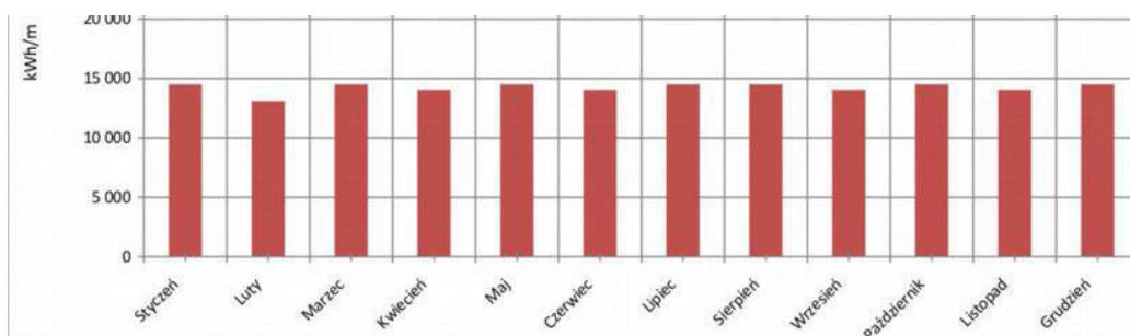
Rys. 10. Przykładowy profil zapotrzebowania na ciepłą wodę użytkową w skali roku.
