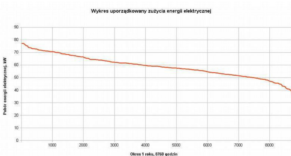
Rys. 7. Wykres uporządkowany poboru mocy elektrycznej w czasie roku w obiekcie basenowym o powierzchni całkowitej 3000 m 2 i powierzchni basenu 312 m 2 .
