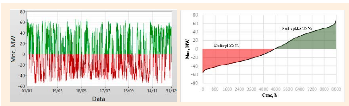
Rys. 30. Bilansowanie przeskalowanego profilu KSE – elektrownie wiatrowe morskie a) profil rocznego bilansu mocy, b) uporządkowany bilans mocy
