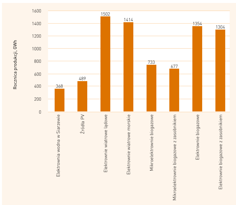
Rys. 16. Porównanie rocznej produkcji w źródłach wytwórczych za 2,2 mld PLN
