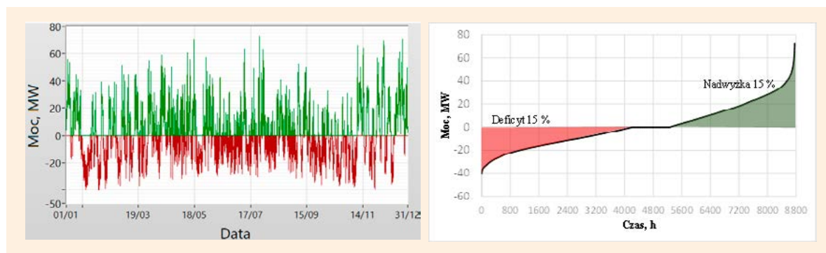
Rys. 39. Bilansowanie przeskalowanego profilu KSE – WME a) profil rocznego bilansu mocy, b) uporządkowany bilans mocy
