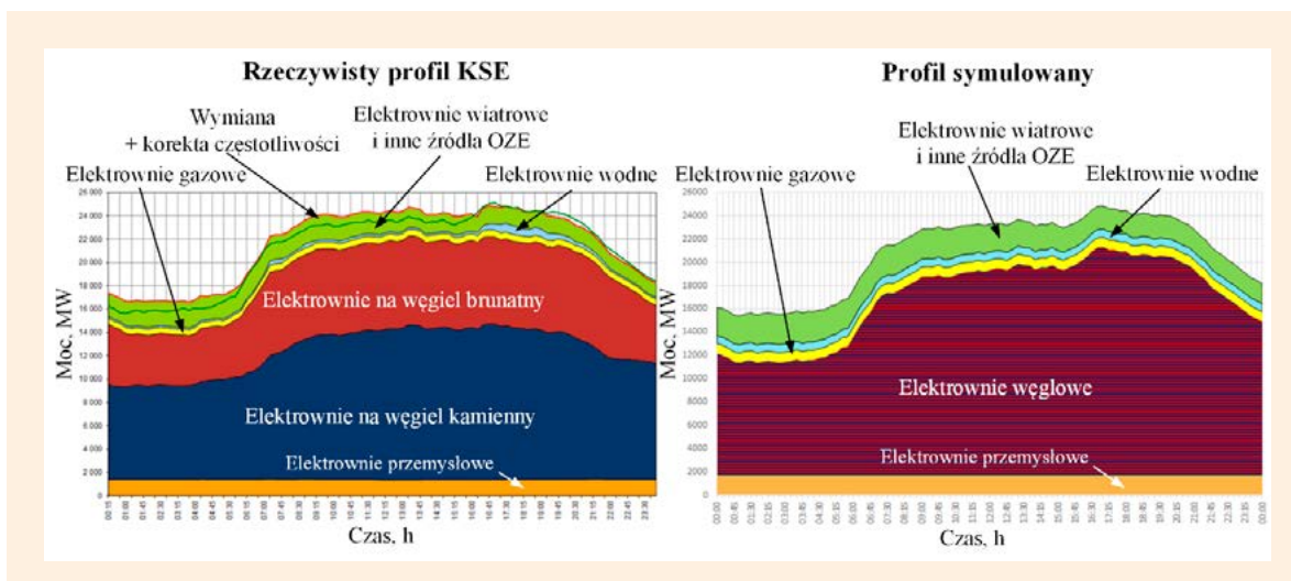
Rys. 5. Porównanie rzeczywistych profili KSE z symulowanymi w dniu największego zapotrzebowania na energię elektryczną 07.01.2015
