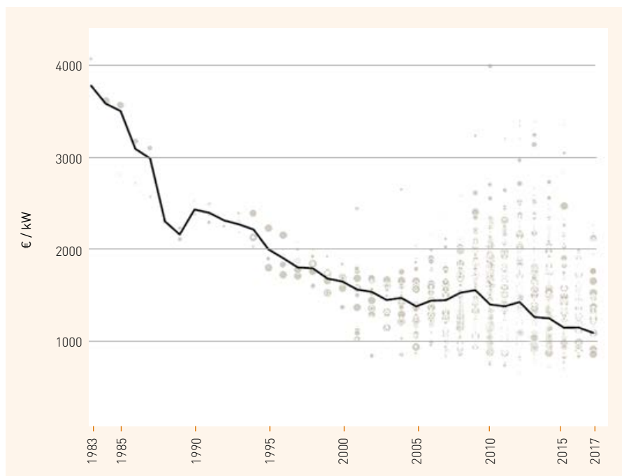
Rys. 17. Nakłady inwestycyjne elektrowni wiatrowych lądowych na przestrzeni lat 1983–2017 w zrealizowanych projektach [18]
