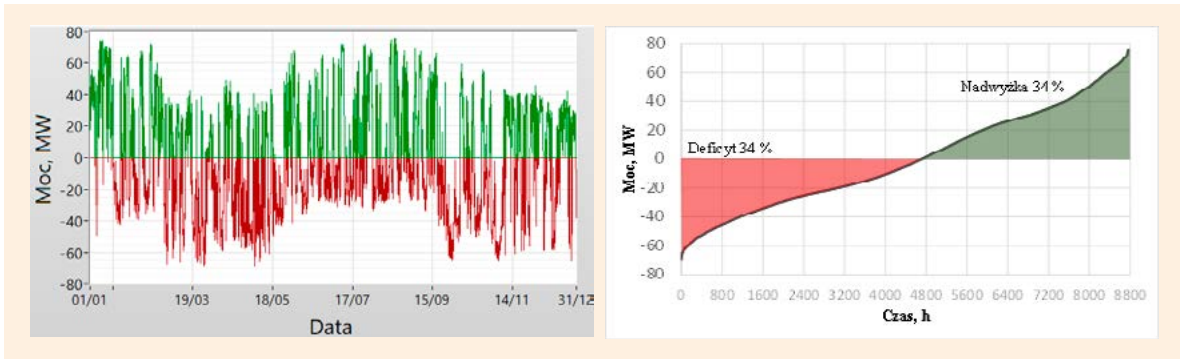
Rys. 31. Bilansowanie profilu elektrowni wodnej w Siarzewie – elektrownie wiatrowe morskie a) profil rocznego bilansu mocy, b) uporządkowany bilans mocy
