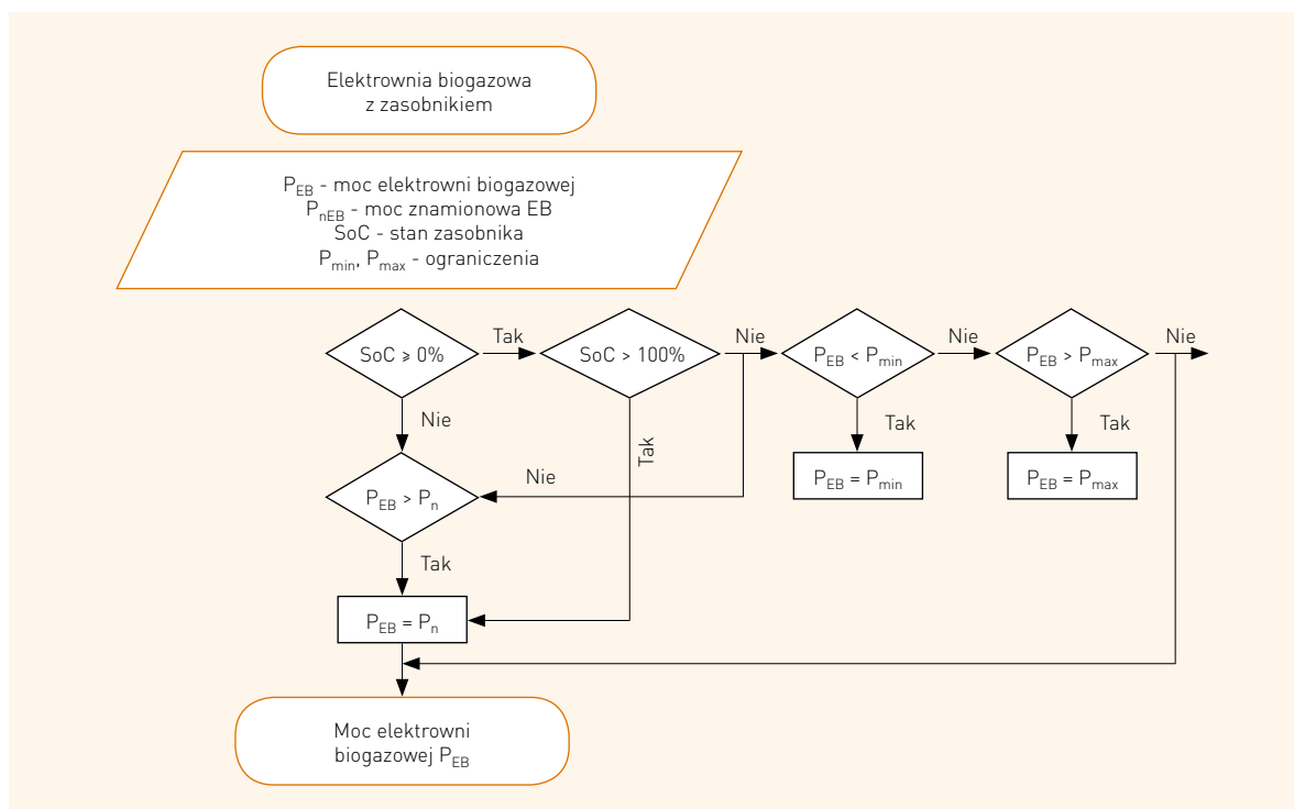
Rys. 1. Algorytm pracy elektrowni biogazowej z zasobnikiem [11]
