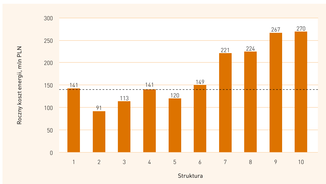
Rys. 20. Roczny koszt energii dla dziesięciu struktur wytwórczych (368 GWh)
