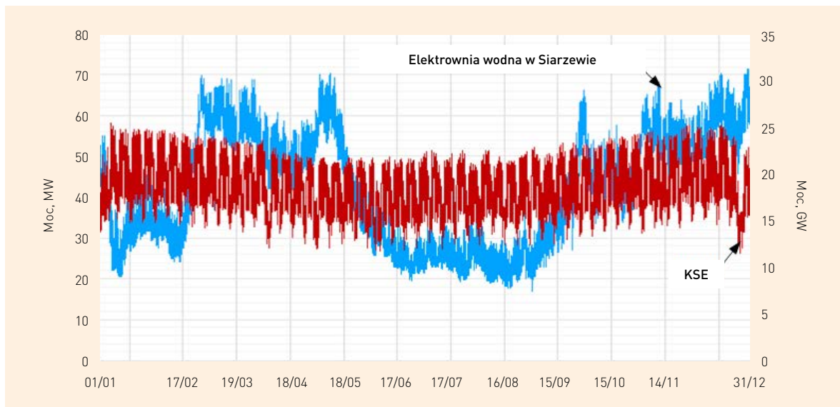
Rys. 6. Przewidywany profil produkcji elektrowni wodnej w Siarzewie oraz profil zapotrzebowania KSE przeskalowany do prognozowanej rocznej produkcji w elektrowni w Siarzewie (368 GWh)
