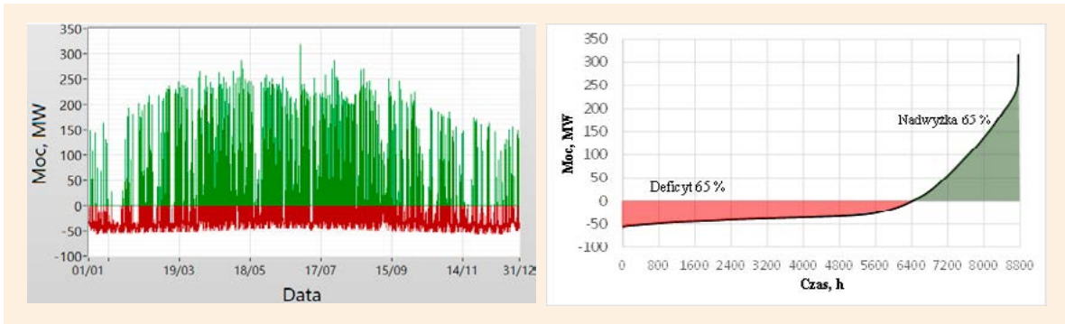
Rys. 22. Bilansowanie przeskalowanego profilu KSE – źródła PV a) profil rocznego bilansu mocy, b) uporządkowany bilans mocy
