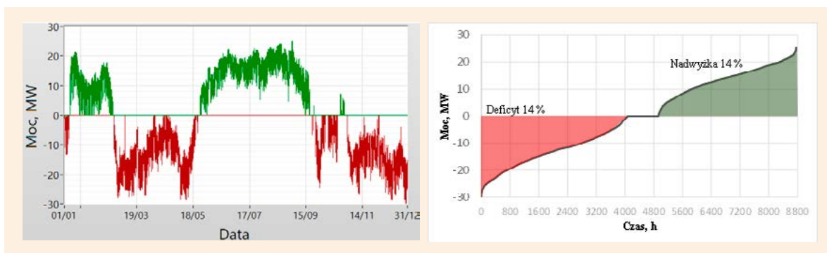
Rys. 35. Bilansowanie profilu elektrowni wodnej w Siarzewie – elektrownie i mikroelektrownie biogazowe z zasobnikiem: a) profil rocznego bilansu mocy, b) uporządkowany bilans mocy
