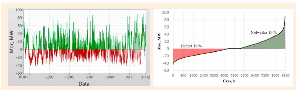
Rys. 26. Bilansowanie przeskalowanego profilu KSE – źródła PV, elektrownie wiatrowe, mikroelektrownie biogazowe z zasobnikiem a) profil rocznego bilansu mocy, b) uporządkowany bilans mocy
