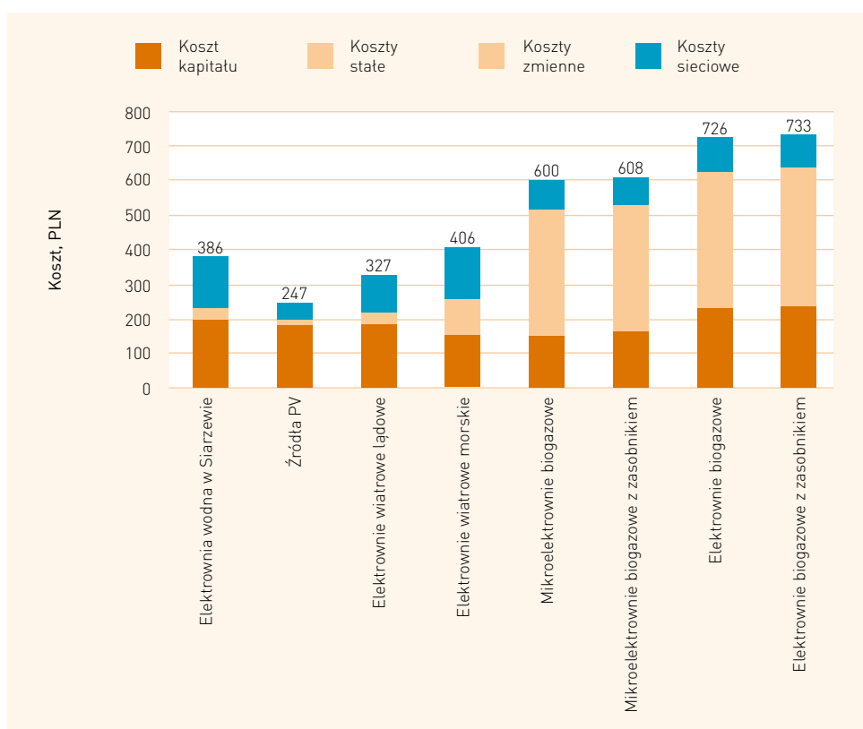
Rys. 19. Struktura kosztów wytwarzania wraz z opłatami sieciowymi wybranych technologii
