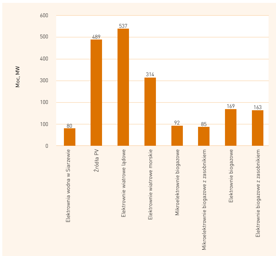
Rys. 15. Porównanie mocy źródeł wytwórczych za 2,2 mld PLN
