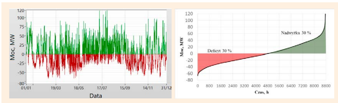
Rys. 25. Bilansowanie profilu elektrowni wodnej w Siarzewie – źródła PV, elektrownie wiatrowe a) profil rocznego bilansu mocy, b) uporządkowany bilans mocy
