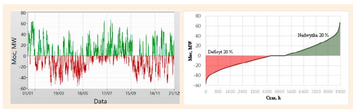
Rys. 40. Bilansowanie profilu elektrowni wodnej w Siarzewie – WME a) profil rocznego bilansu mocy, b) uporządkowany bilans mocy
