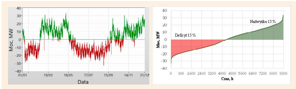
Rys. 21. Bilansowanie przeskalowanego profilu KSE – Elektrownia Wodna Siarzewo a) profil rocznego bilansu mocy, b) uporządkowany bilans mocy
