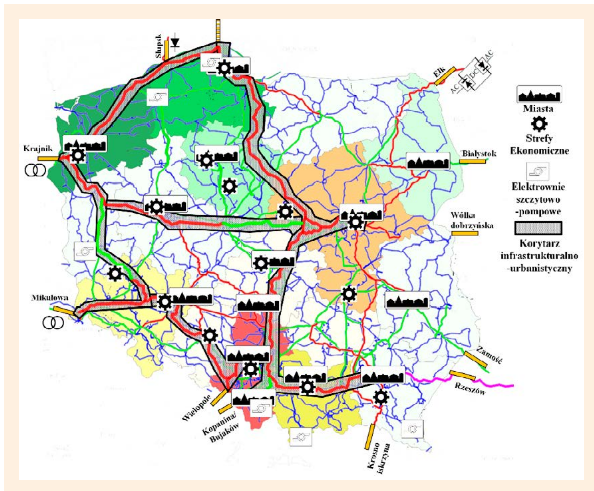
Rys. 12. Hybrydowe (AC-DC) dostępne korytarze przesyłowe, otwierające polskim strefom/korytarzom urbanistycznym dostęp do północnoeuropejskich zasobów wiatrowych offshore (Morze Północne, Baltyk) i skandynawskich (Norwegia, Szwecja) wodnych zasobów magazynowych [10]
