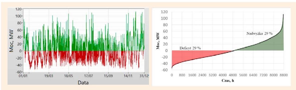
Rys. 24. Bilansowanie przeskalowanego profilu KSE – źródła PV, elektrownie wiatrowe a) profil rocznego bilansu mocy, b) uporządkowany bilans mocy
