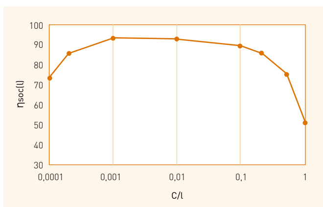
Rys. 2. Zależność sprawności ładowania akumulatora od parametru C/I [4, 5]
