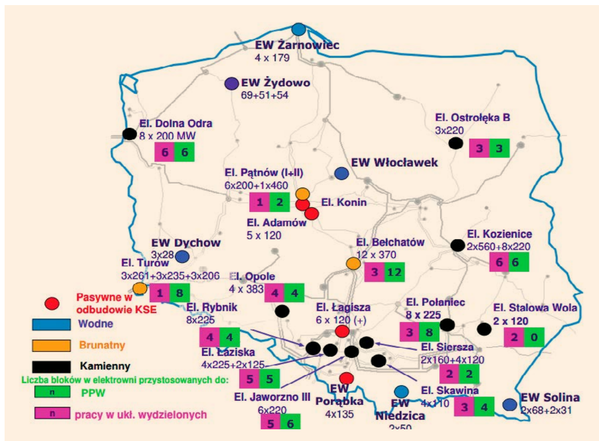
Rys. 41. Elektrownie systemowe KSE w planie obrony i odbudowy systemu (PSE-Operator) [5]
