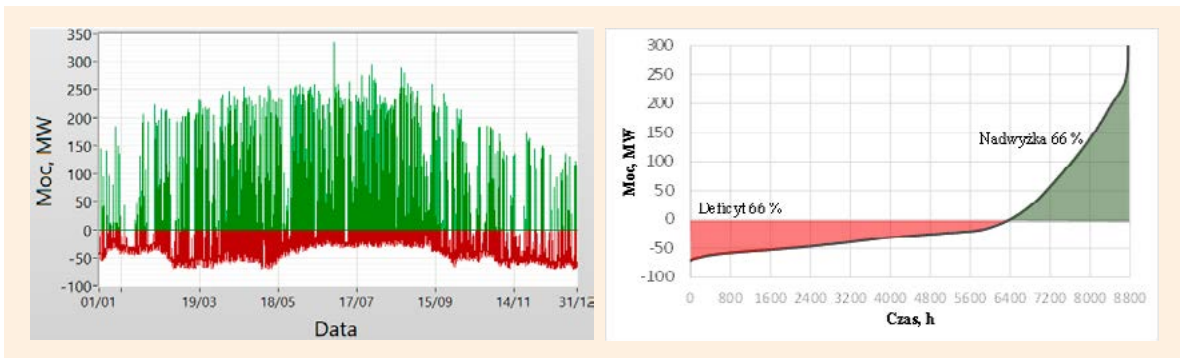
Rys. 23. Bilansowanie profilu elektrowni wodnej w Siarzewie – źródła PV a) profil rocznego bilansu mocy, b) uporządkowany bilans mocy
