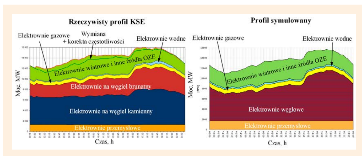
Rys. 4. Porównanie rzeczywistych profili KSE z symulowanymi w dniu najmniejszego zapotrzebowania na energię elektryczną 26.12.2015
